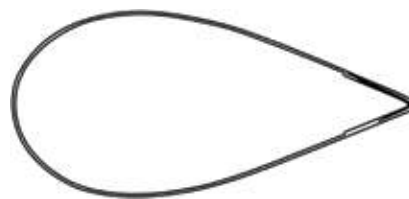
446300FX Tonsil Wire Loops , closed, pack of 100 pcs., Ø 0.4 mm, length 50 mm Tonsillenschlingen , geschlossen, Packung zu 100 Stück, Ø 0,4 mm, Länge 50 mm
