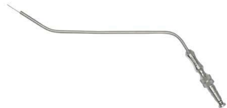
111710FX Suction Tube by Kahn-Frazier , slightly curved, malleable shaft, WL 15 cm, 10 Fr. Saugrohr nach Kahn-Frazier , leicht gebogen, biegsamer Schaft, NL 15 cm, 10 Charr.
